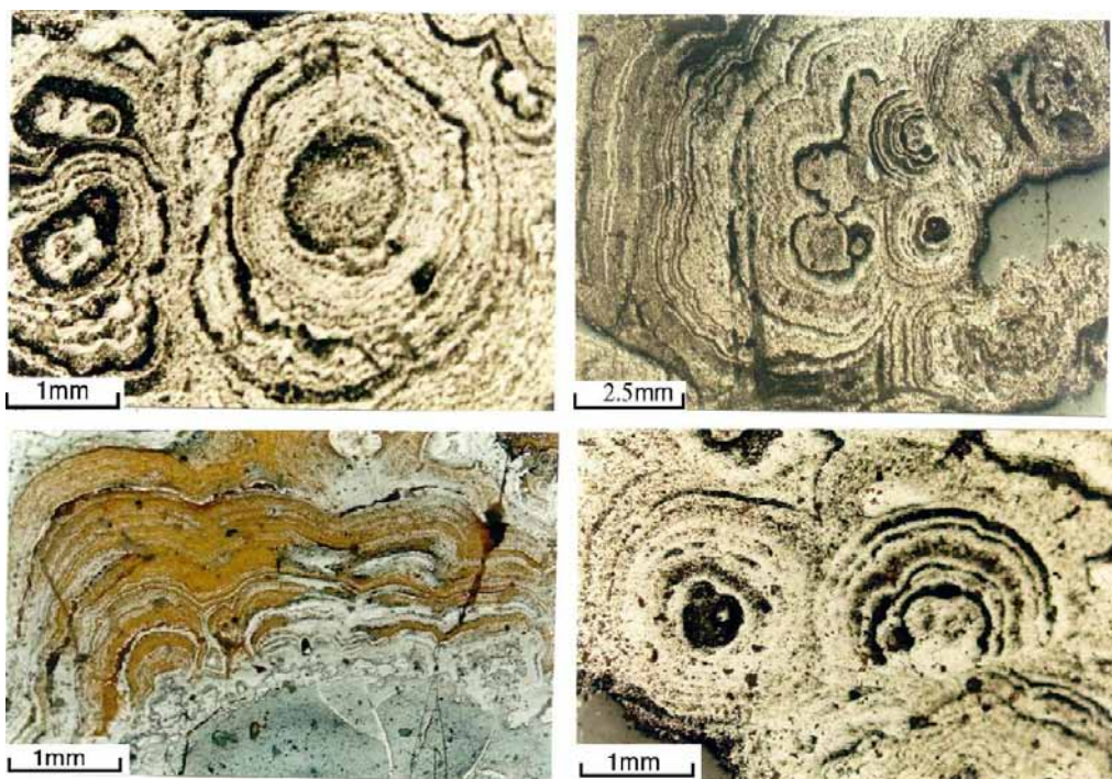
شکل ۶- بافت کلوform، نواربندی هم‌مرکز و رشد کروی پیزولیتی در مقاطع صیقلی کانه پیرولولزیت. نور بازتابی.
