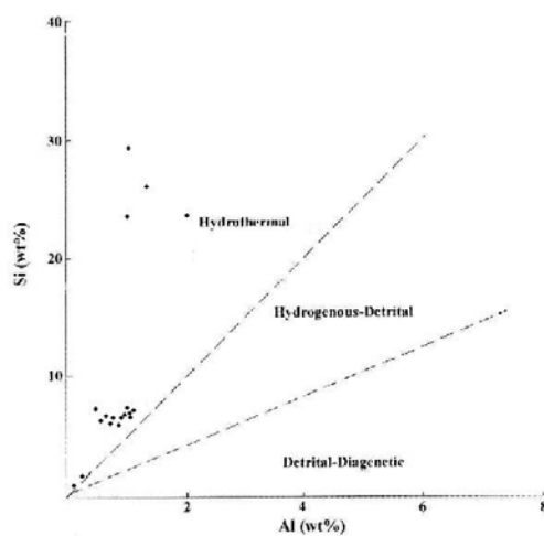
شکل ۸- نمودار Si-Al و تفکیک فرایندهای مختلف تشکیل نهشته‌های فرومگنز (Crerar et al., 1982).
