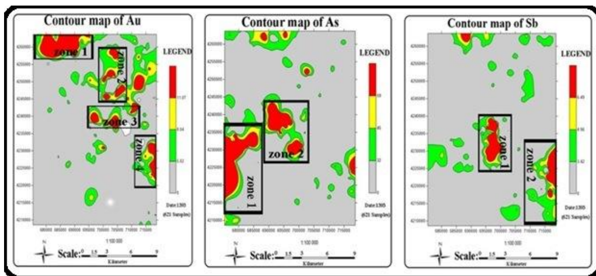
شکل ۸- نقشه کنتری هم‌مقدار شیمیایی عنصر طلا، آرسنیک و آنتیموان در منطقه اهر
