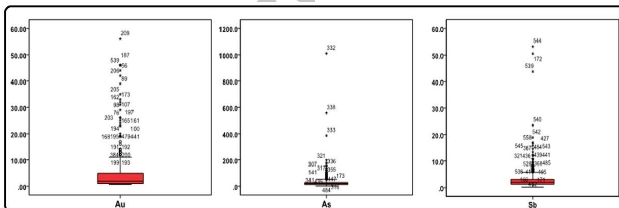
شکل ۵- نمودار جعبه ای عناصر طلا، آرسنیک و آنتیموان
