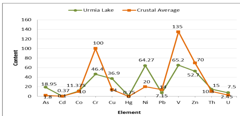
شکل ۲- نمودار مقایسه غلظت فلزات سنگین و عناصر رادیواکتیو در رسوبات و نمک‌های دریاچه ارومیه با مقادیر متوسط پوستانه‌ای (۸).
