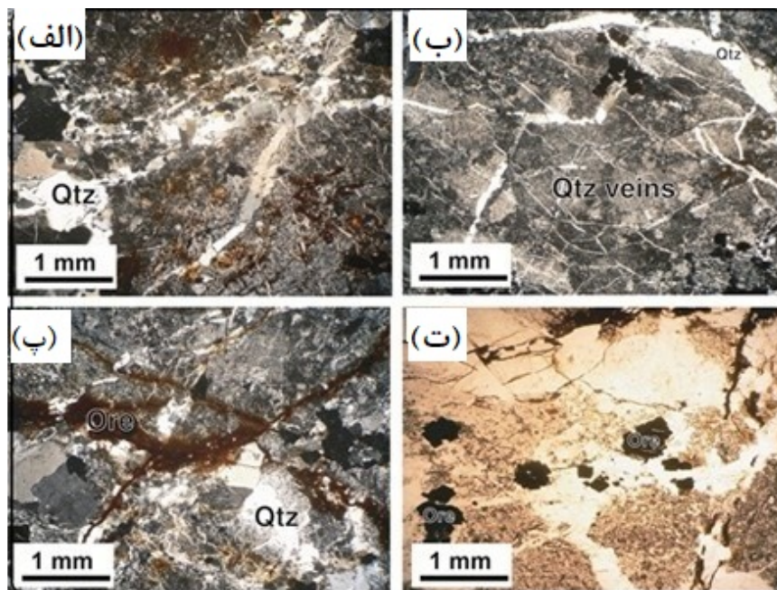
شکل ۱۲ تصاویر میکروسکوپی از دگرسانی سیلیسی در واحد آندزیت: (الف) رگچه‌های کوارتز و کلسیت، (ب) مقدار زیادی دانه‌های پراکنده و رگچه کوارتزی، (پ) رگچه ماده معدنی در سنگ دگرسان و (ت) بلورهای شکل‌دار پیریت.
