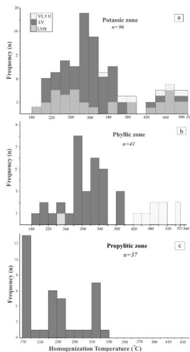
شکل ۱۲: فراوانی دماهای همگن شدن میانبارهای سیال برای رگچه‌های کوارتزی زون‌های دگرسانی: a: پتاسیک، b: فلیک، c: پروپیلیتیک.
