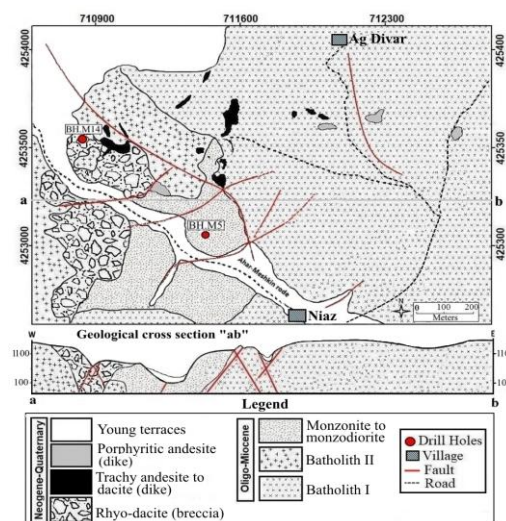
شکل ۱: نقشه زمین‌شناسی محدوده مورد مطالعه با نمایش واحدهای سنگی به تفکیک سن و نمایش محل دو گمانه حفاری BH.M5 و BH.M14.
