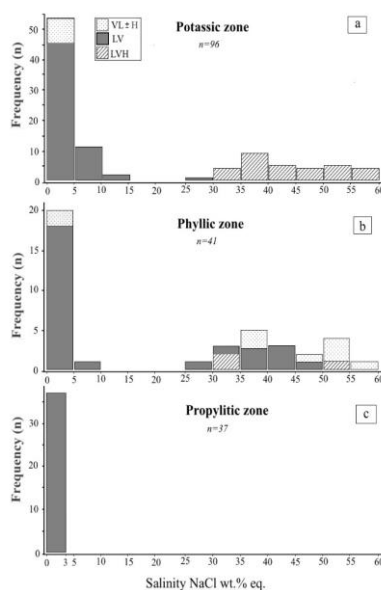
شکل ۱۳: فراوانی شوری میانبارهای سیال برای زون‌های دگرسانی، a: پتاسیک، b: فلیک، c: پروپیلیتیک.
