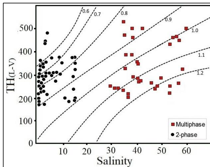
شکل ۱۴: نمودار دمای همگن شدن/ شوری جهت تعیین چگالی سیالات درگیر به تفکیک انواع دو فازی و چند فازی ( Zhang and Frantz, 1987). بیشتر نمونه‌های دو فازی در بازه ۰/۶۲-۰/۸۷ و میانبرهای چند فازی در بازه ۰/۹-۱/۲ قرار می‌گیرند.
