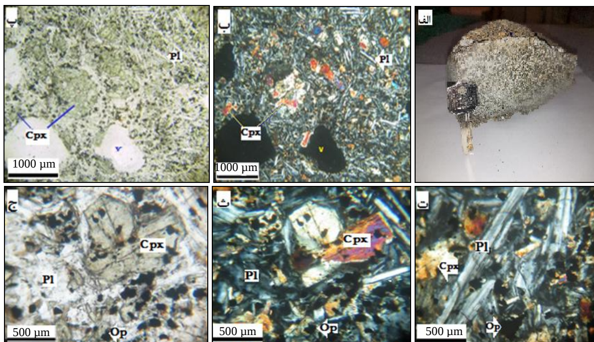
شکل 3. تصاویر ماکروسکوپی و میکروسکوپی از واحد بازالتی در منطقه یارالوجه (نور ppl و xpl). (الف) نمونه دستی برش خورده بازالت، ب و پ) فنوکریست های پلاژیوکلاز، کلینوپیروکسن و میکرولیت های پلاژیوکلاز، (ت و ث) پلاژیوکلاز های شکل دار و کلینوپیروکسن های نیمه شکل دار همراه کانی های اپک، (ث و ج) پلاژیوکلاز ها و کلینوپیروکسن های دارای منطقه بندی نوسانی که متحمل دگرسانی شده و همراه اپک. (Pl = پلاژیوکلاز؛ Cpx = کلینوپیروکسن؛ Op = اپک (تیره)) [7].
