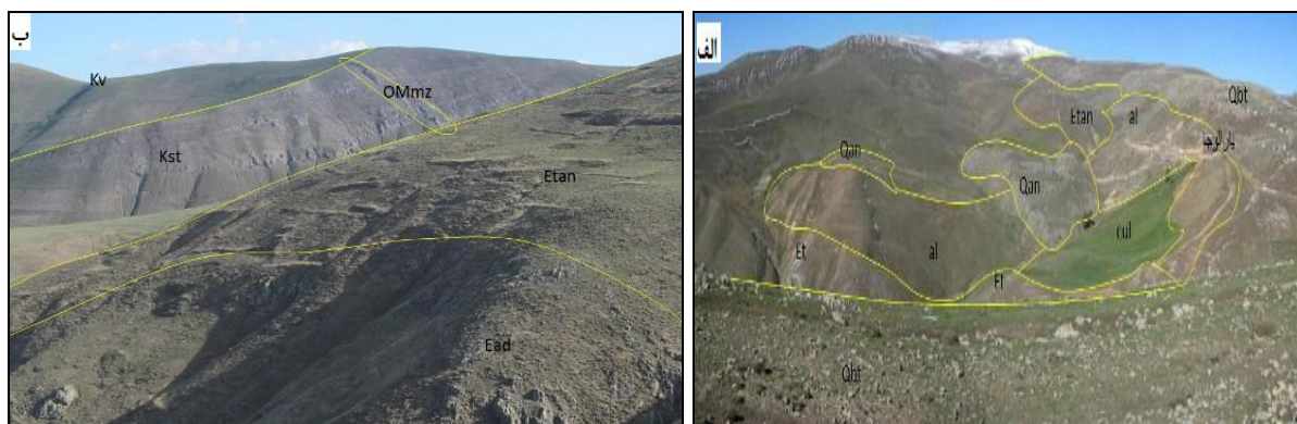
شکل 2. تصاویر صحرایی از منطقه یارالوجه. الف) محدوده یارالوجه شرقی، ب) محدوده یارالوجه غربی.
