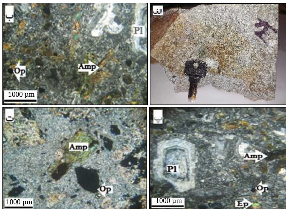
شکل ۴. تصاویر ماکروسکوپی و میکروسکوپی از واحد آندزیتی در منطقه یارالوجه (نور xpl). الف) نمونه دستی برش خورده آندزیت، ب و پ) کانی‌های پلاژیوکلاز، آمفیبول و اپیک که دچار دگرسانی فیلیک شده اند، ت) کانی‌های غیر دگرسانی واحد آندزیتی. (Pl = پلاژیوکلاز؛ Cpx = کلینوپیروکسن؛ Op = تیره؛ Ep = اپیدوت).
