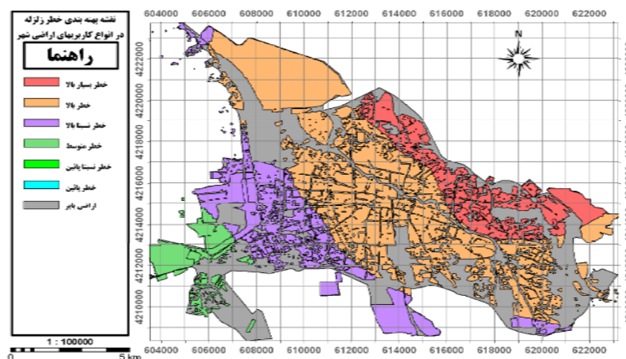
شکل ۶: نقشه‌ی پهنه‌بندی خطر زلزله در کاربری اراضی شهر تبریز مأخذ: روستایی، ۱۳۸۵
