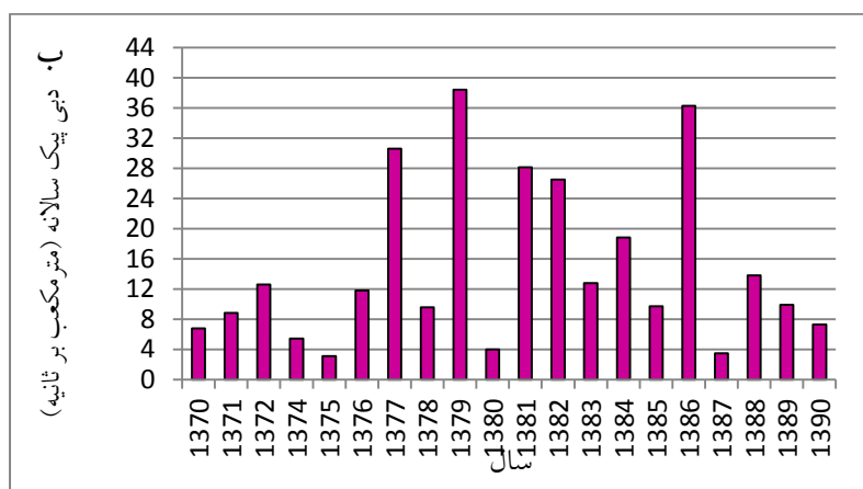
شکل ۱۱: حداکثر دبی سالانه حوضه آبریز لیقوان طی دوره آماری ۱۳۷۰-۱۳۹۰ (الف: ایستگاه لیقوان، ب: ایستگاه هروی)
