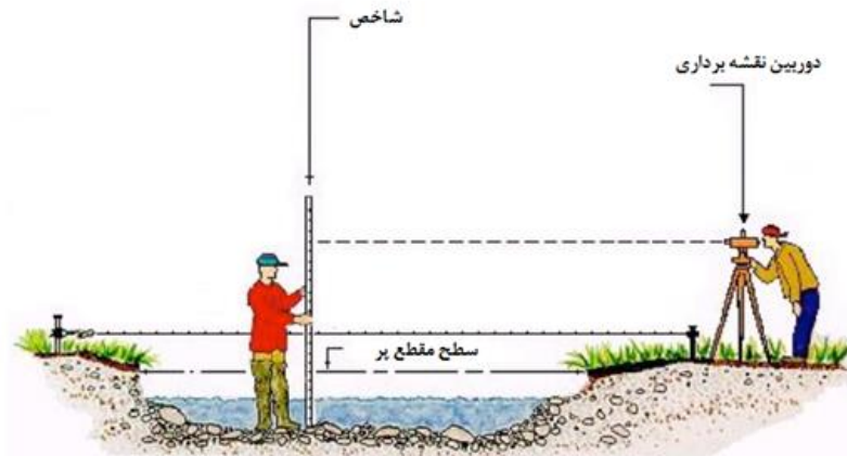
شکل ۲: سطح مقطع پر در یک مقطع عرضی اصلاح شده از راسگن ۱۹۹۶ (آربلیز و همکاران ۳۴ ، ۲۰۰۷: ۱۹۱)
