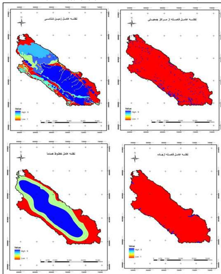
نقشه های شماره ۹، ۸، ۷، ۶: کلاسه بندی شده عوامل موثر در بروز ناپایداری های دامنه ای بینالود
