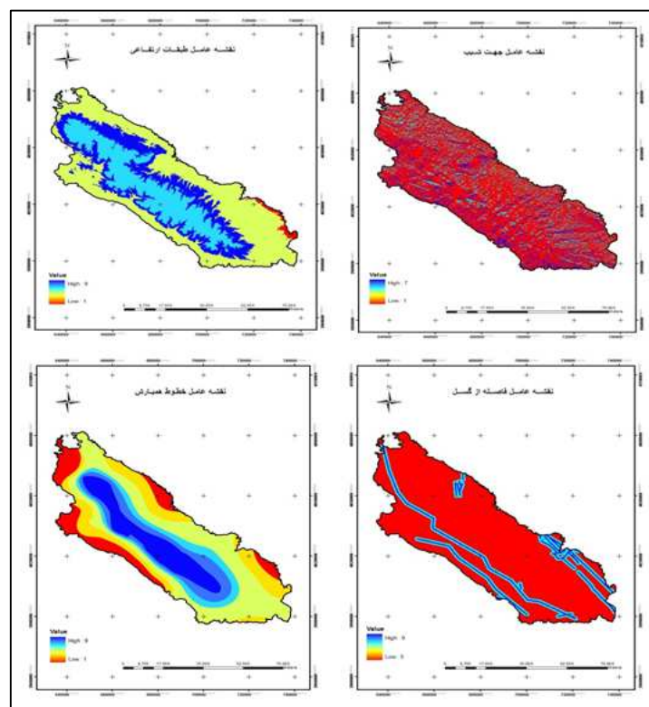
نقشه شماره ۵، ۴، ۳، ۲: عوامل کلاسه بندی شده موثر در بروز ناپایداری های دامنه ای
