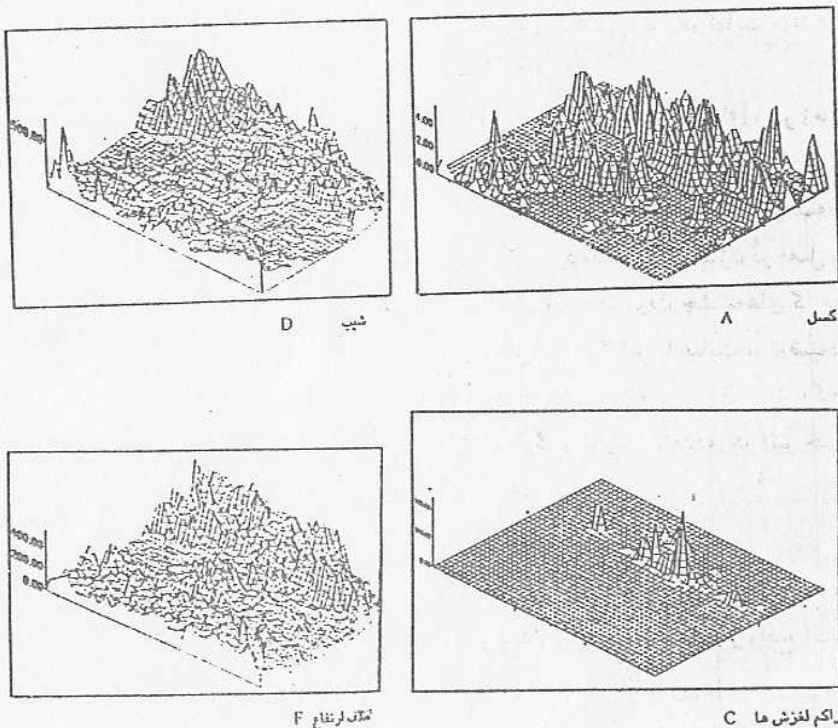
شکل ۳- بلوک دیاگرام‌های مربوط به تراکم متغیرهای انتخابی (خطی، ۱۳۷۶)
