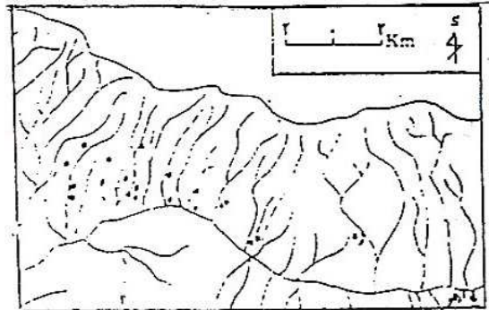
شکل شماره ۱- پراکندگی و علل وقوع لغزشهای دره‌ای
