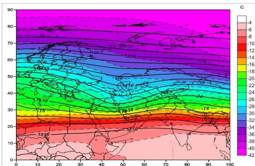
شکل ۳: الگوی ترکیبی دما و ارتفاع تراز ۵۰۰ خوشه اول
