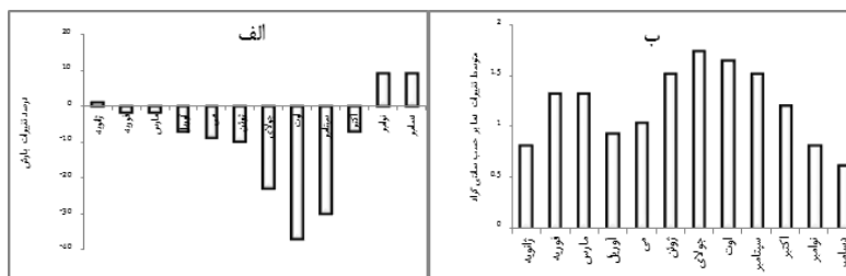
شکل ۴- تغییرات پیش بینی شده برای بارش (الف) و دما (ب) برای دوره ۲۰۱۳-۲۰۳۰ نسبت به دوره مبنا در حوضه آبریز تسوج با استفاده از مدل HADCM۳ و سناریوی A۲
