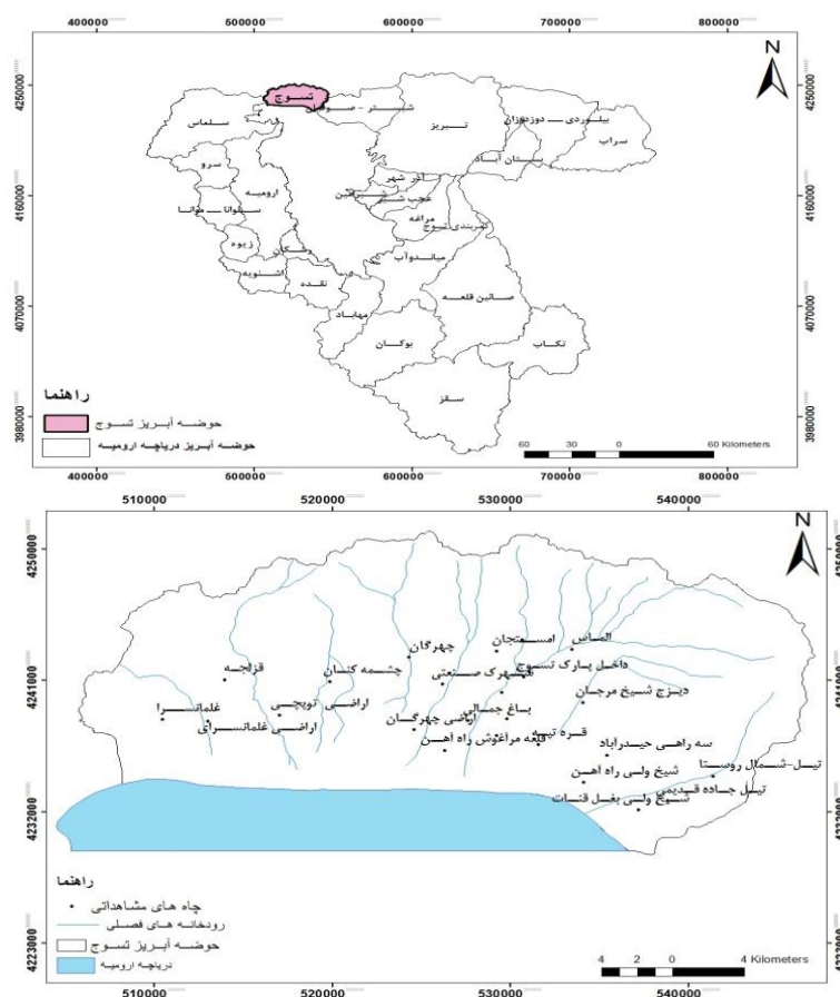
شکل ۱- موقعیت منطقه مورد مطالعه
