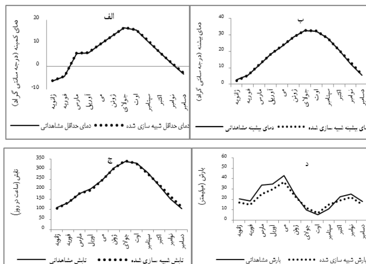
شکل ۲- مقایسه مقادیر نتایج حاصل از مدل و دیده بانی شده برای دماهای کمینه (الف)، بیشینه (ب)، تابش (ج) و بارش (د) در حوضه آبریز تسوج (۱۹۸۴-۲۰۱۲)
