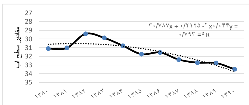
شکل ۴: هیدروگراف سالانه آب زیرزمینی دشت مرند (سال‌های ۹۰-۱۳۸۰)
