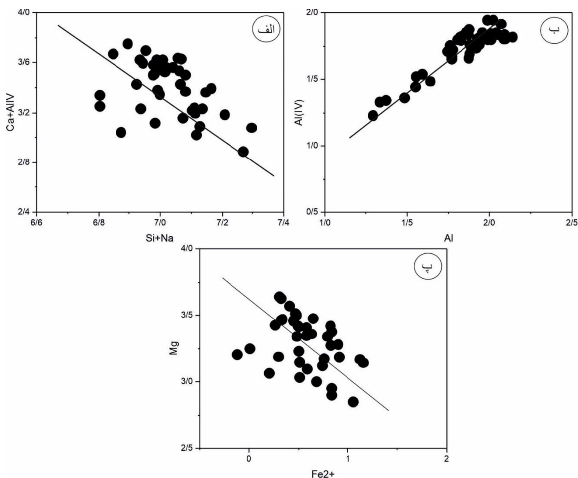
شکل ۷ الف) نمودار Si+Na نسبت به Ca+Al_{IV} [۱۳]، ب) نمودار (Al_{IV}) نسبت به Al^{IV} که بر اساس آن، آمفیبول‌های تجزیه شده دارای روند خطی هستند [۱۱]، پ) نمودار Fe^{2+} نسبت به Mg .
