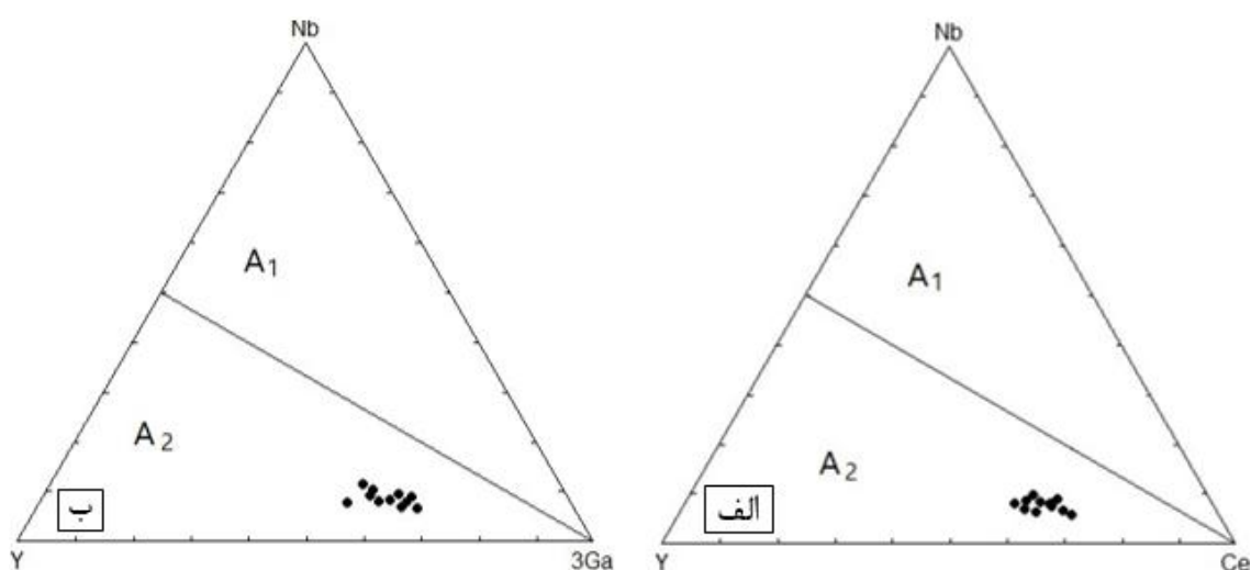
شکل ۱۲ الف- نمودار مثلثی Y-Nb-Ce و ب- نمودار مثلثی Y-Nb-3Ga برای تفکیک محیط زمین ساختی گرانیت‌های نوع A به دو نوع A_1 و A_2 [۹] که سنگ‌های مورد بررسی بر آنها جایابی شده‌اند.
