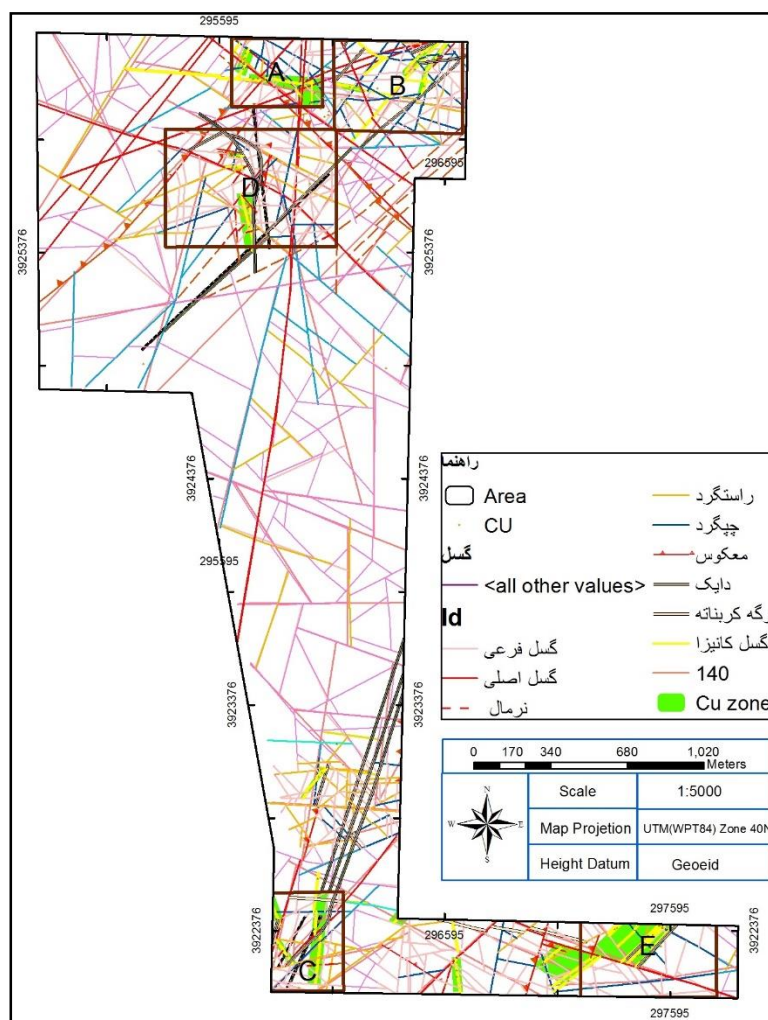
شکل ۴. نقشه ی ساختاری منطقه و زون های کانی زا
