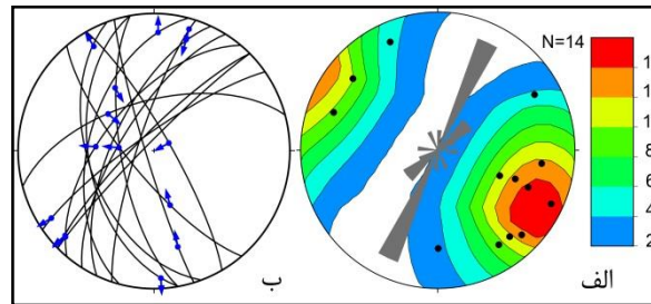
شکل ۶: الف) موقعیت قطب دایک‌ها. نمودار گل سرخی، نشانگر امتداد دایک‌ها است. ب) موقعیت صفحات گسلی قبل از کانه‌زایی. پیکان‌ها نشانگر جهت حرکت فرادیواره نسبت به فرودیواره گسل هستند.
