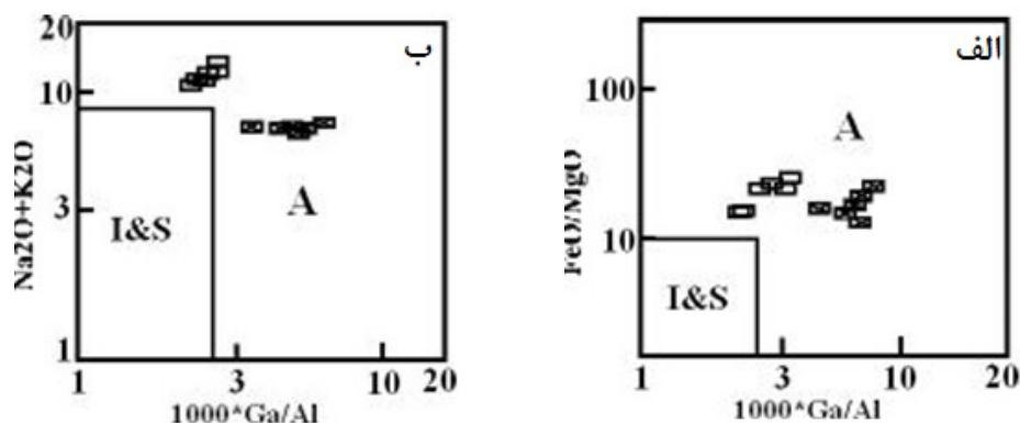
شکل ۷ نمودارهای دوتایی الف) FeO/MgO نسبت به 1000*Ga/Al و ب) Na_2O+K_2O نسبت به 1000*Ga/Al و جایگاه نمونه‌های مورد بررسی بر آنها [۲۴] (نشانه‌ها مانند شکل ۴)
