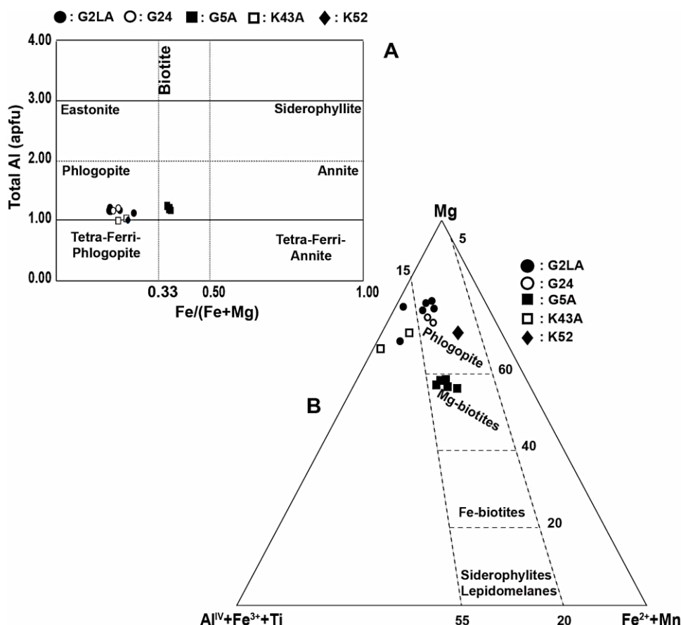
شکل ۴: الف) نمودارهای Fe/(Fe+Mg) در مقابل Al_T (apfu) برگرفته از ریدر و همکاران (۱۹۹۸) جهت نام‌گذاری بیوتیت‌ها قرارگیری نمونه‌های بیوتیتی در کمپلکس آتشفشانی-نفوذی سارای در آن. ب) نمودار مثلی Mg - (Al^{IV}+Fe^{3+}+Ti)-(Fe^{2+}+Mn) برگرفته از فوستر (۱۹۶۰) و قرارگیری نمونه‌های بیوتیتی آتشفشان سارای در آن.
