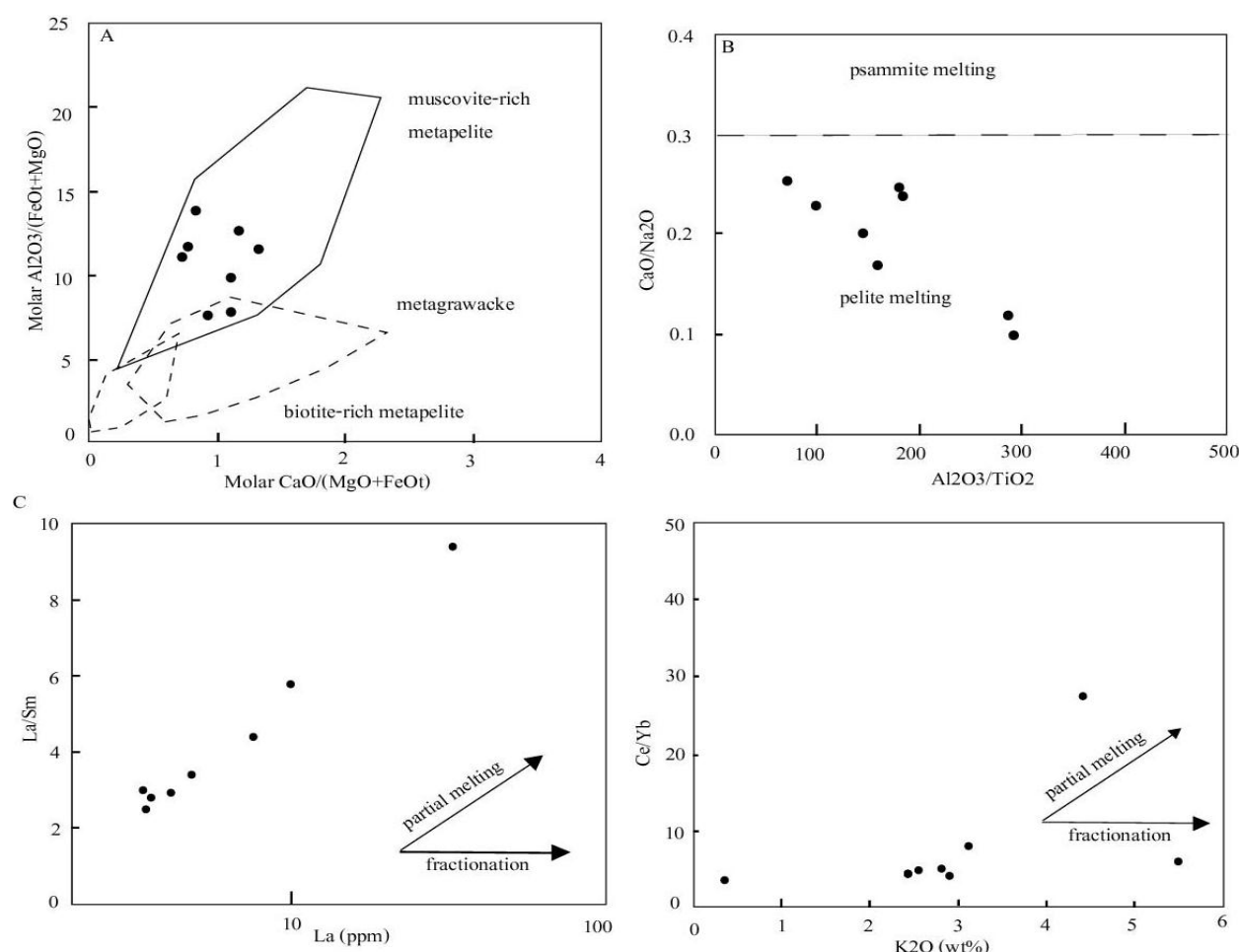
شکل ۹- مسکوویت گرانیات ها و آلکالی فلدسپار گرانیات های گرمی چای در: (A) نمودار CaO/(FeO+MgO+TiO_2) در برابر Al_2O_3/(FeO+MgO) برای رسوب های دگرگون شده (Patiño Douce, 1999)؛ (B) نمودار Al_2O_3/TiO_2 در برابر CaO/Na_2O که نشان دهنده مذاب های تجربی پدید آمده از رسوب های سمیتی و پلیتی است (Jung and Pfänder, 2007)؛ (C) نمودار La/Sm در برابر La (Patiño Douce, 1999)؛ (D) نمودار K_2O در برابر Ce/Yb (Jung and Pfänder, 2007) (دو نمودار C و D نشان دهنده نقش فرایند ذوب بخشی در پیدایش گرانیات S هستند؛ هر چند نقش تفریق را نمی توان نادیده گرفت. گرانیات تیپ A زیر گروه A1 به شمار می رود)
