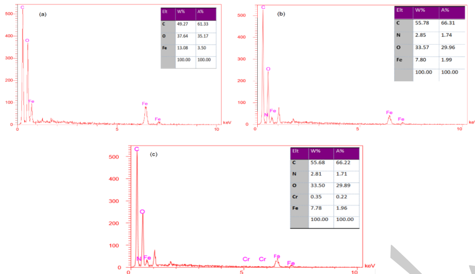
Fig. 4. EDX analysis of: a) MGO, b) MGO-IDA before Cr ion adsorption and c) MGO-IDA after Cr ion adsorption شکل ۴- نتایج آنالیز EDX: (a) اکسید گرافن مغناطیسی شده، (b) اکسید گرافن مغناطیسی عامل دار شده با ایمینو دی استیک اسید و (c) اکسید گرافن مغناطیسی عامل دار شده با ایمینو دی استیک اسید بعد از جذب کروم
