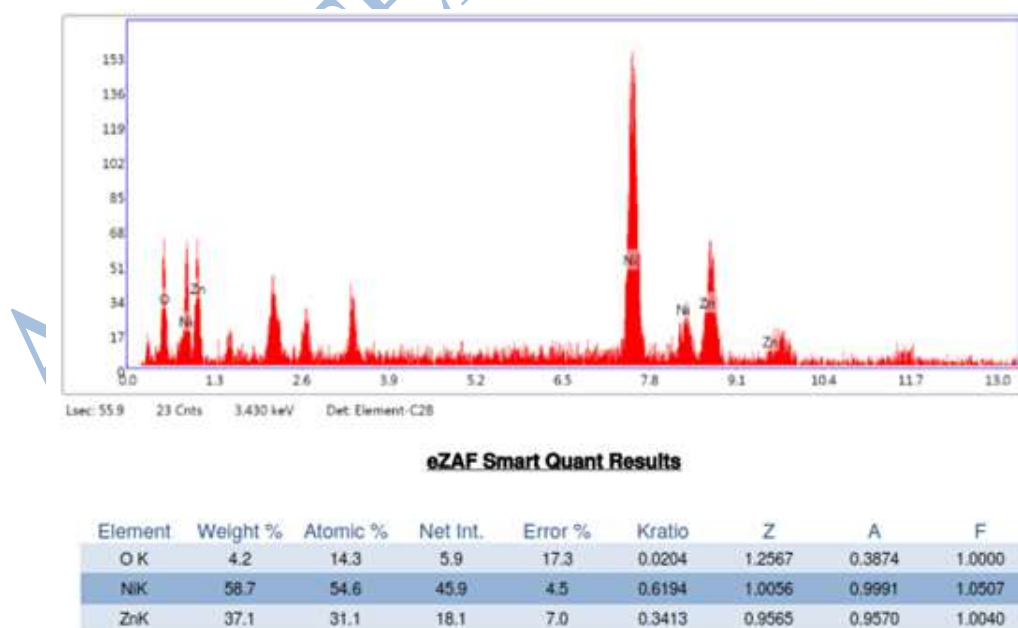
شکل ۳. آنالیز EDS نانوکامپوزیت \text{ZnO}/\text{NiO}
