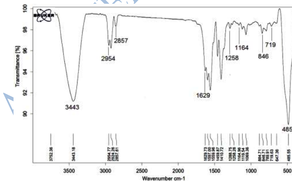
شکل ۵. طیف FTIR حاصل بارگذاری داروی ایبوپروفن روی نانوکامپوزیت ZnO/NiO
