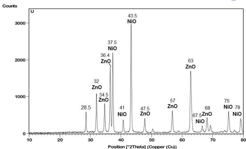
شکل ۱. الگوی XRD نانوکامپوزیت ZnO/NiO تهیه شده با روش هم-رسوبی با عامل پوشاننده عصاره نعنای و عامل بازی کننده NaOH
