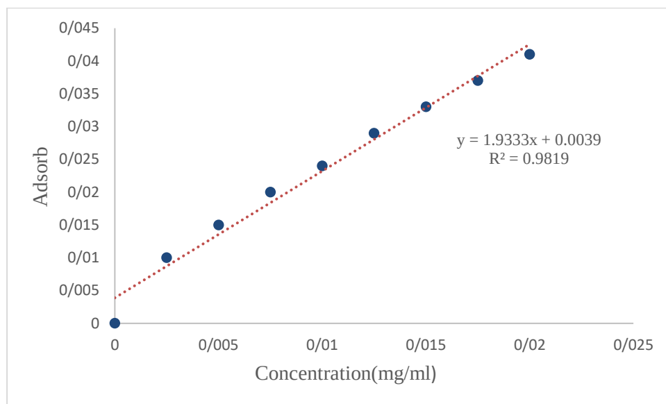
شکل ۶. نمودار کالیبراسیون داروی ایبوپروفن خالص
