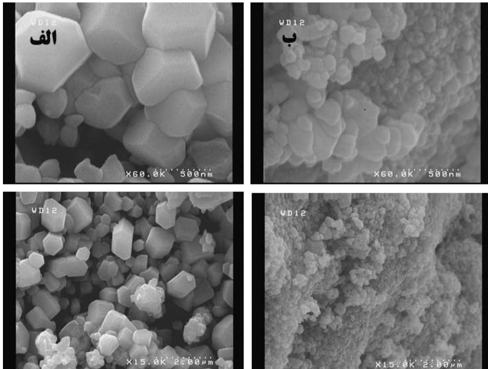
شکل ۲. تصویر SEM نانوکامپوزیت \text{ZnO}/\text{NiO} تهیه شده با روش هم رسوبی با عامل پوشاننده عصاره نعناع و عامل بازی کننده (الف) آمونیاک، (ب) \text{NaOH}
