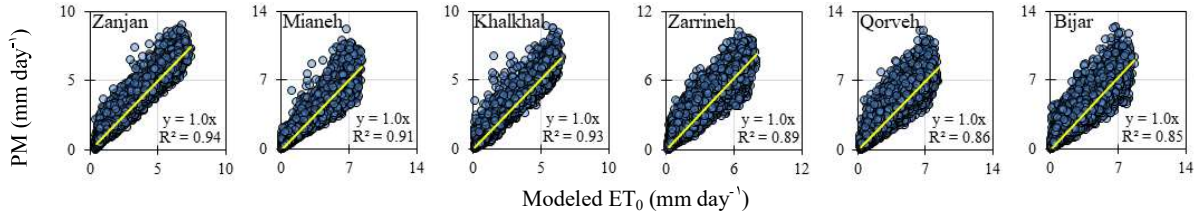
شکل ۳. نمودار پراکنش نقاط محاسباتی ET_0 با معادله FAO56-PM و مقادیر تخمین زده شده با مدل‌های منتخب در ایستگاه‌های مورد مطالعه (پس از واسنجی)
