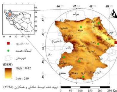
شکل ۱. منطقه مورد مطالعه و ایستگاه‌های منتخب به همراه مدل رقمی ارتفاعی ۱ حوضه آبریز قزل اوزن
