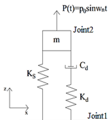
شکل ۴. شماتیک مدل جرم-فنر-میراگر مورد بررسی توسط ترابی
